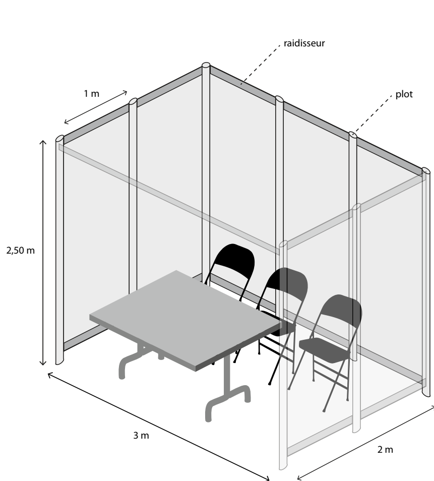
Schéma d'un stand modèle « Standard » (2m x 3m)
